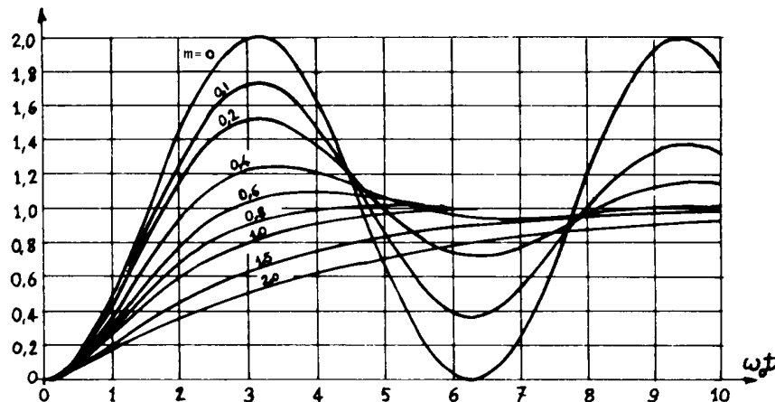
réponse indicielle
